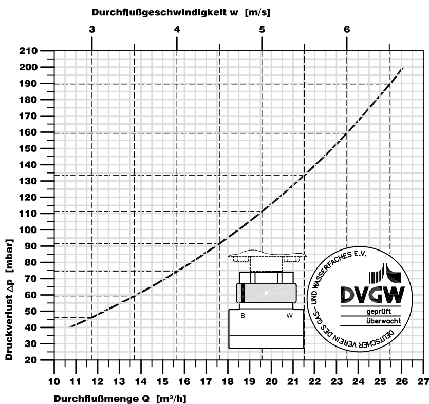
Diagramm Durchflußkennwerte Systemdoppelanschluß
