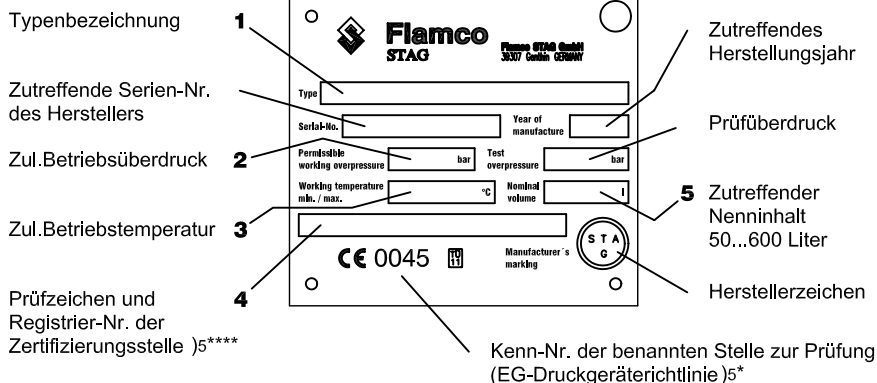
Bild 1 Typenschild
